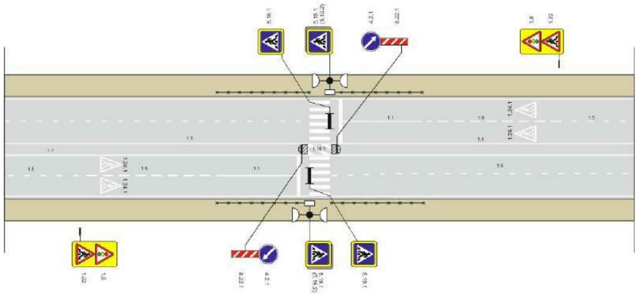
Рисунок Д.10 – Установка ТСОДД в зоне регулируемого пешеходного перехода на участке дороги с четырьмя полосами и более с разделительной полосой
