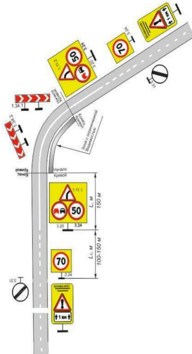
Рисунок Д.16 – Применение ТСОДД на участках дорог с двумя полосами с горизонтальными кривыми и ограниченной видимостью:
