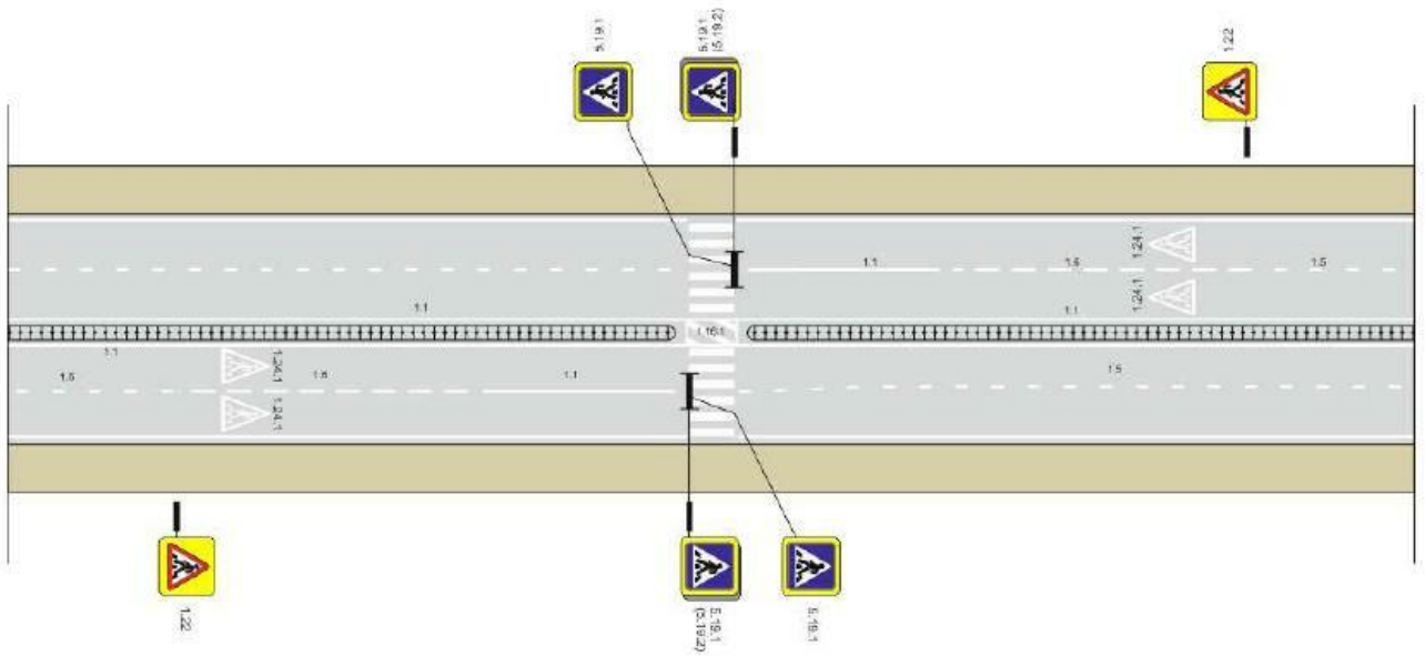
Рисунок Д.6 – Установка ТСОДД при обустройстве нерегулируемого пешеходного перехода
