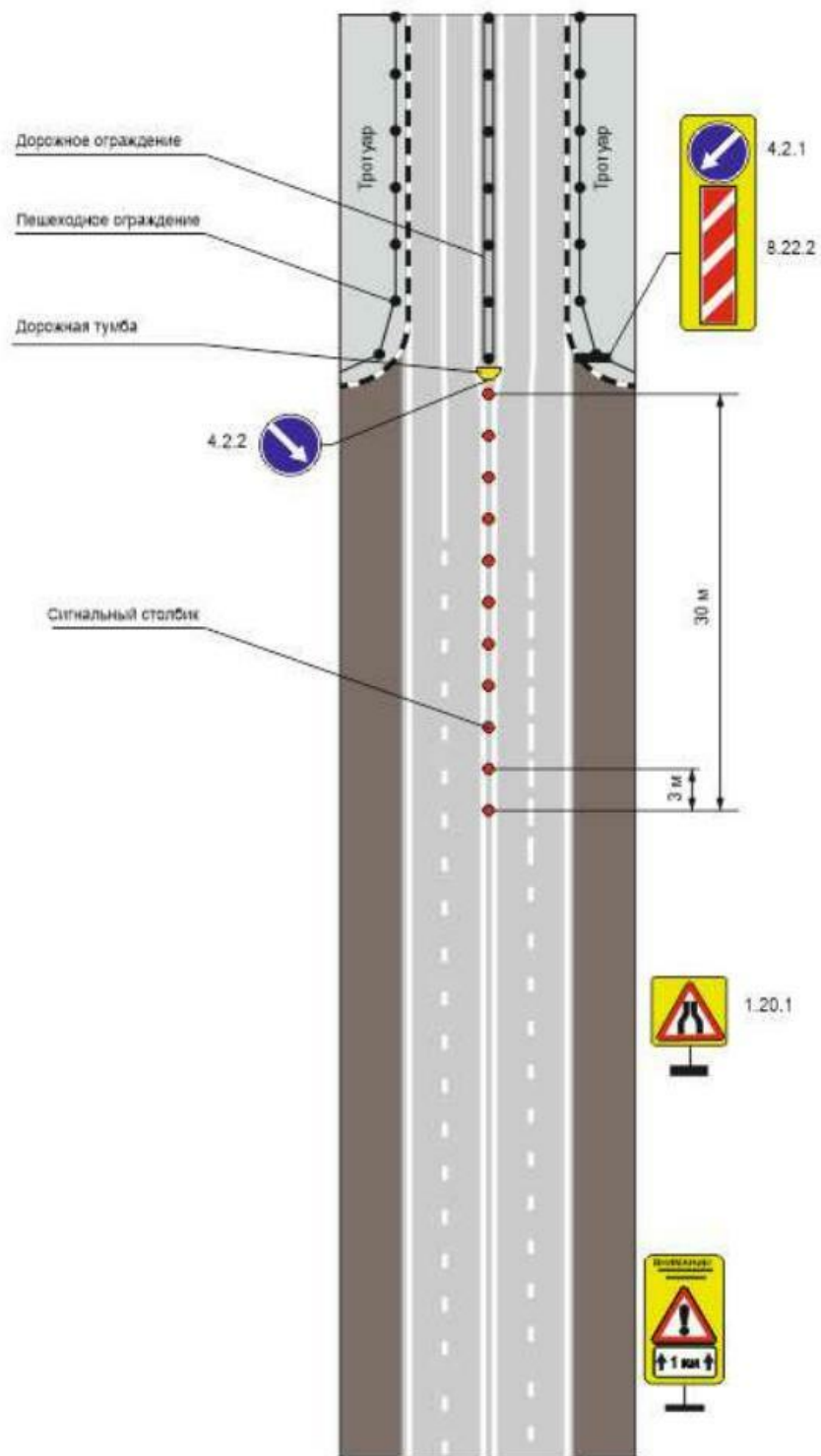
Рисунок Д.21 – Размещение ТСОДД на опасных участках дорог в местах сужения проезжей части
